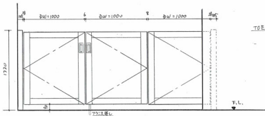
外観図
