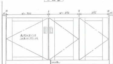
外観図
